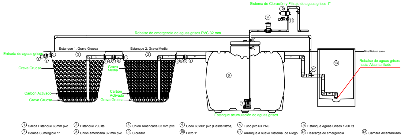
VISTA LATERAL ESTANQUES FILTRADORES AGUAS GRISES
