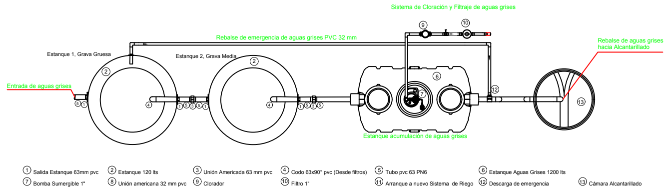
VISTA PLANTA ESTANQUES FILTRADORES AGUAS GRISES
