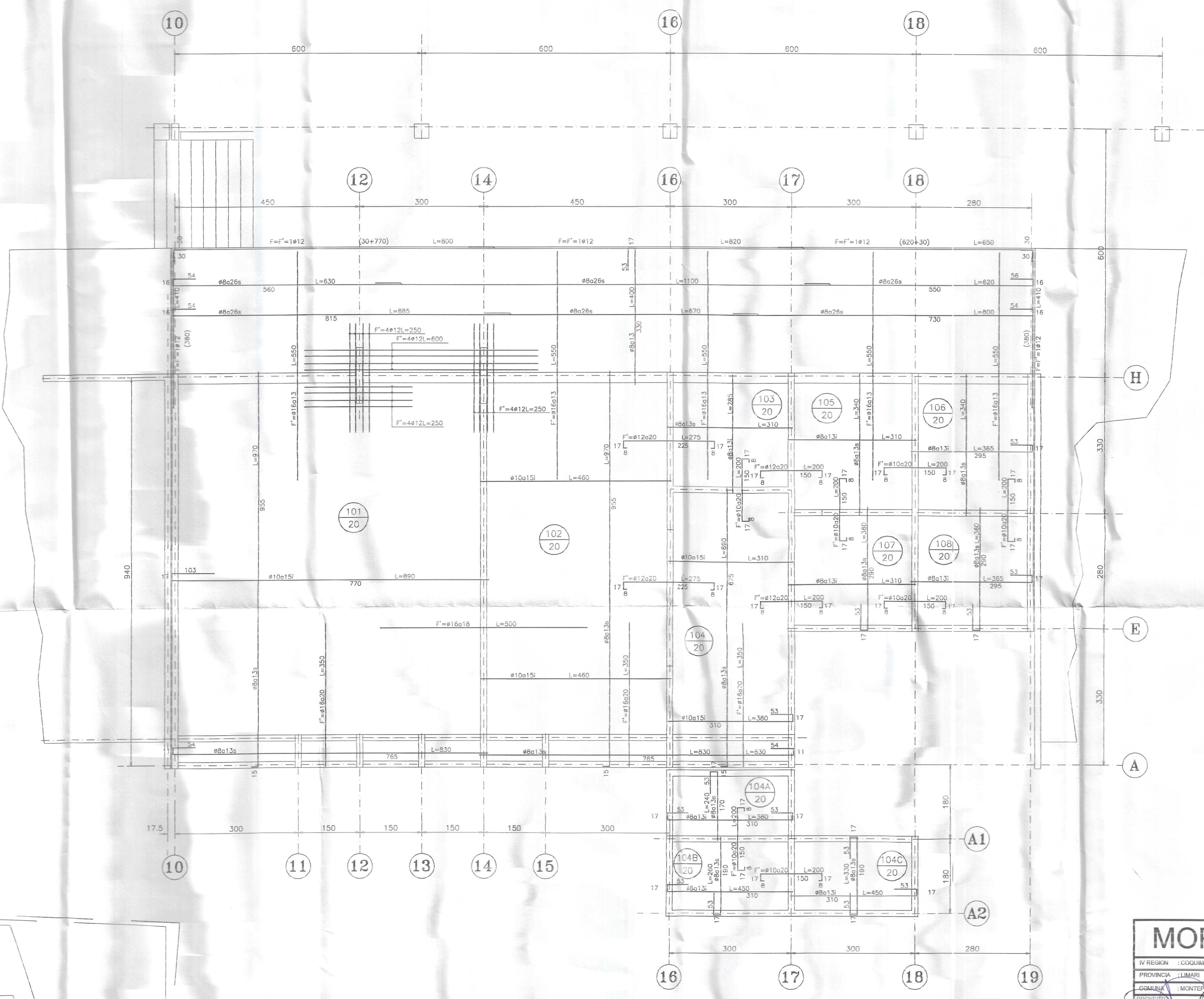
PLANTA DE LOSAS 1º PISO ESCALA 1:50
