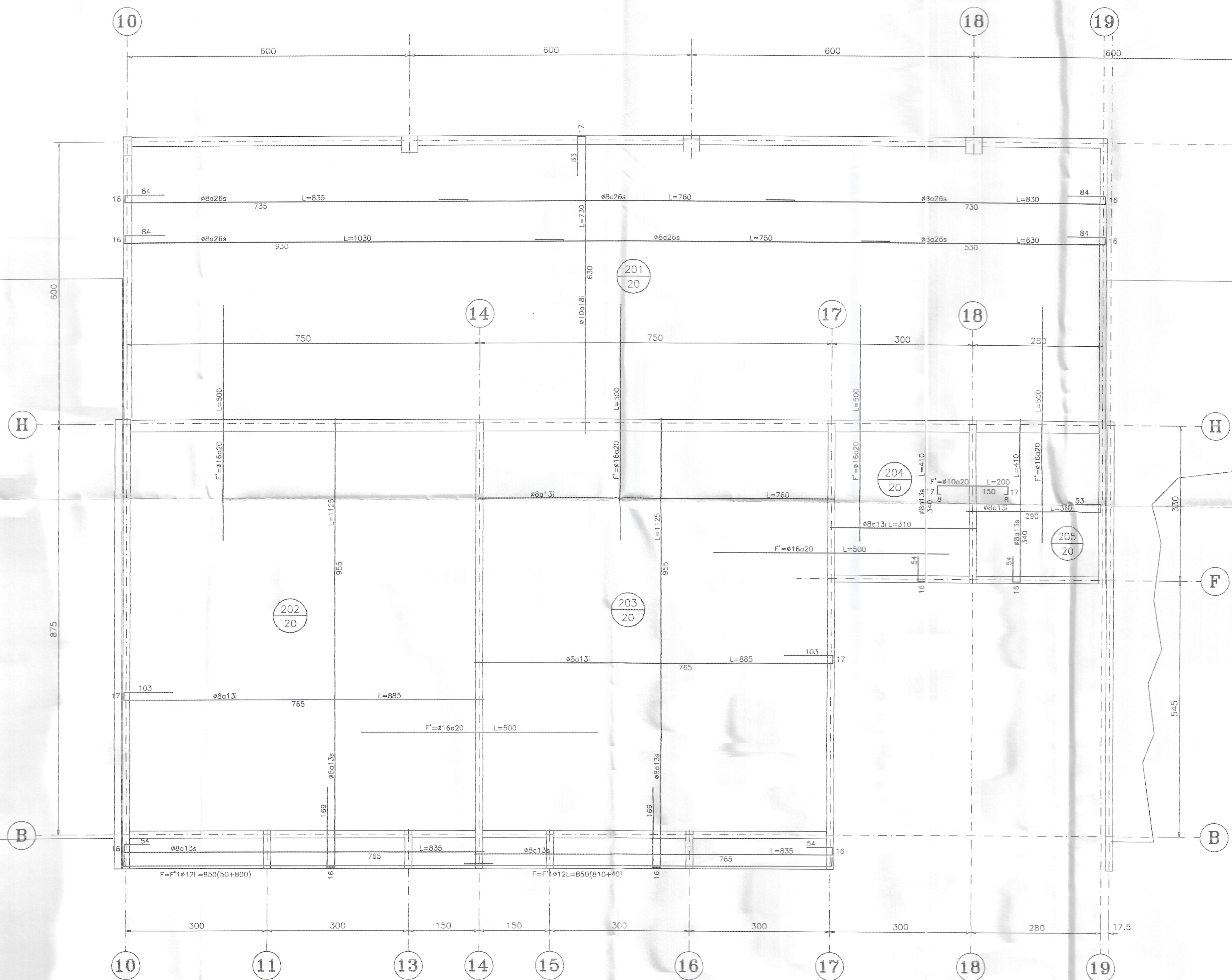
PLANTA DE LOSAS 2º PISO ESCALA 1:50
