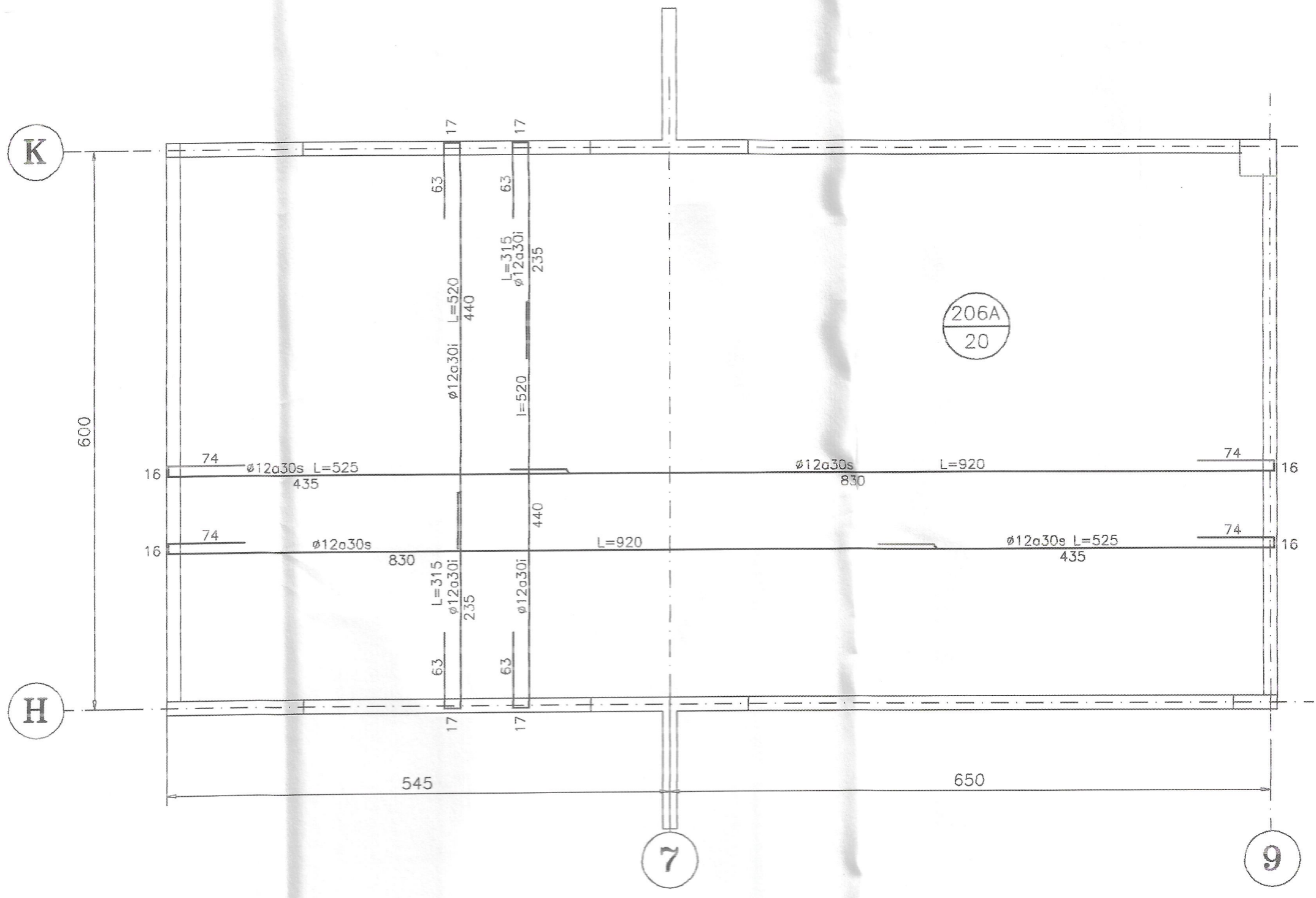
PLANTA Nv. +102.29 ESCALA 1:50
