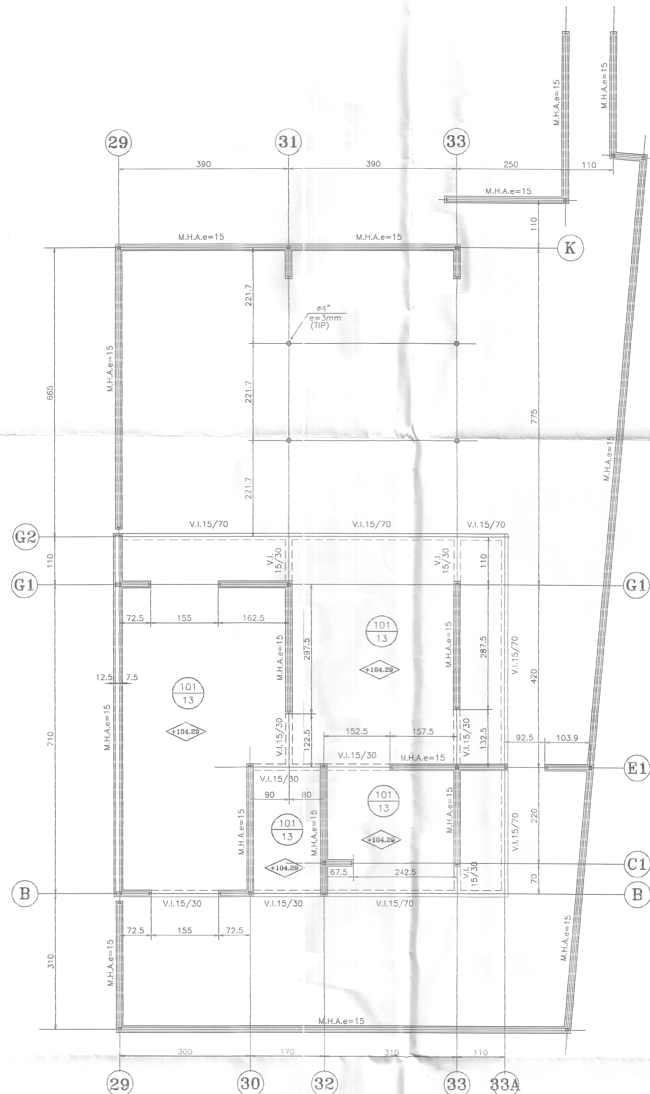
(CASA DEL DIRECTOR) PLANTA DE ESTRUCTURAS 1ºPISO ESCALA 1:50
