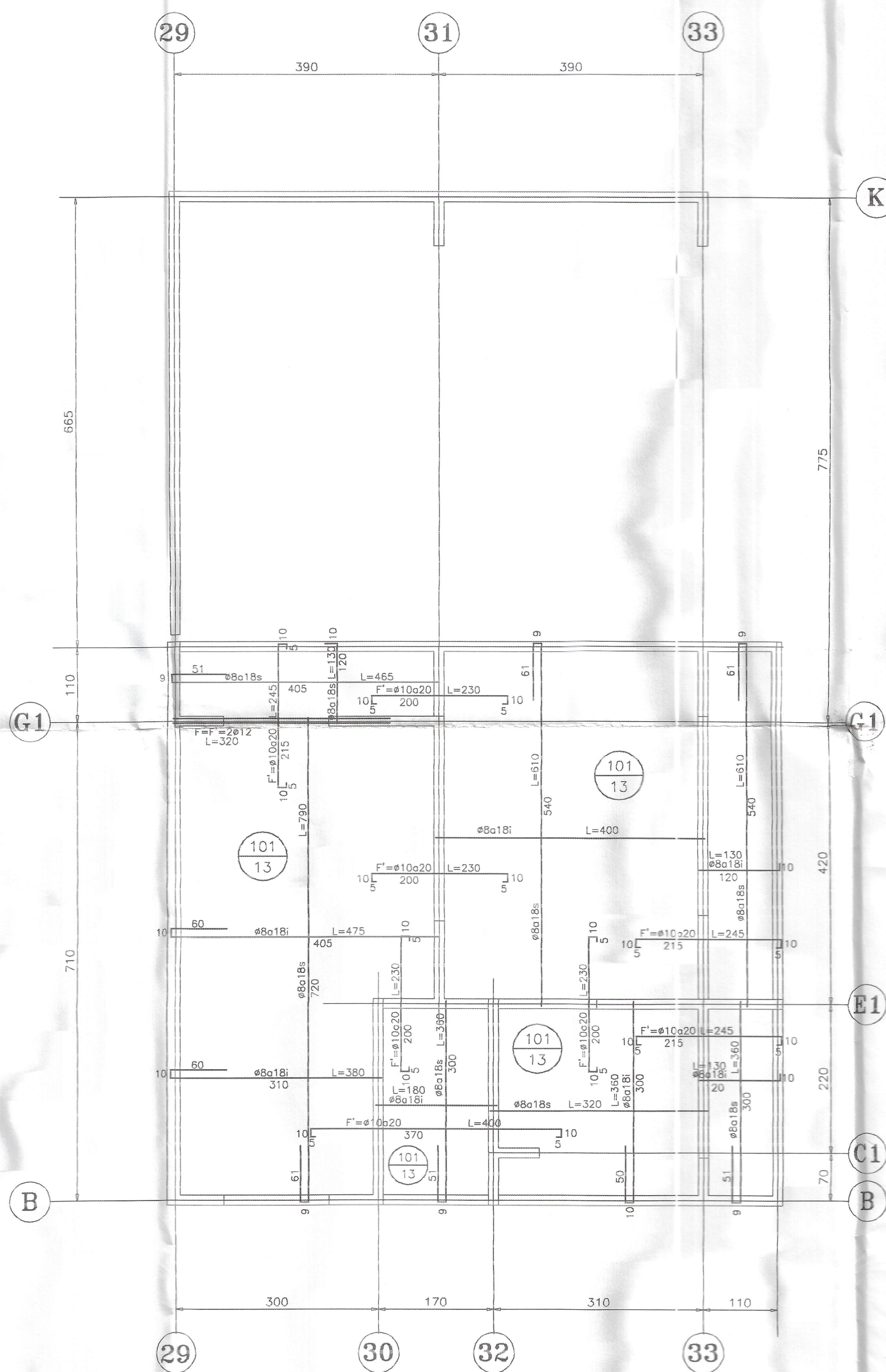
(CASA DEL DIRECTOR) PLANTA DE LOSAS 1ºPISO ESCALA 1:50
