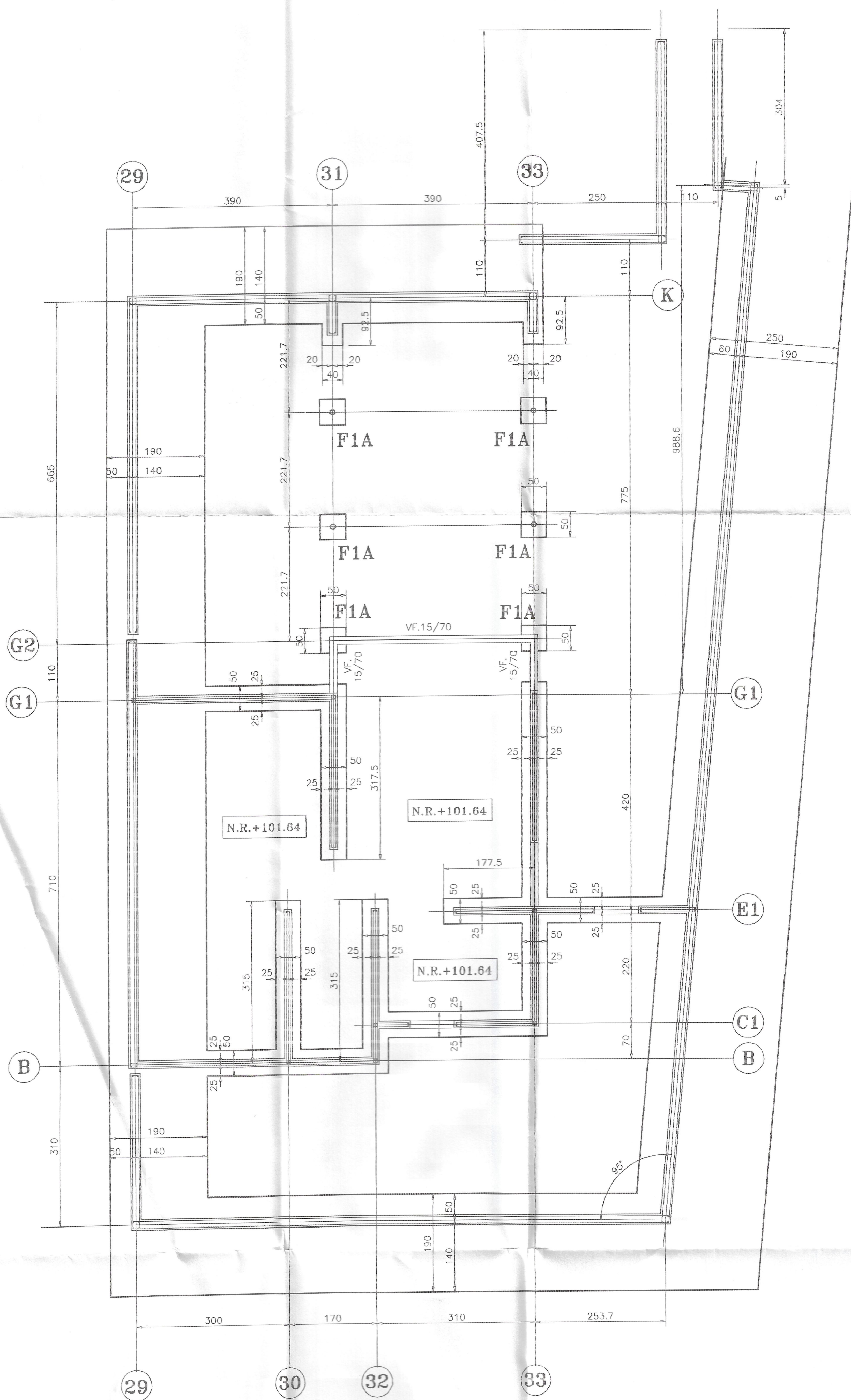
(CASA DEL DIRECTOR) PLANTA DE FUNDACIONES ESCALA 1:50
