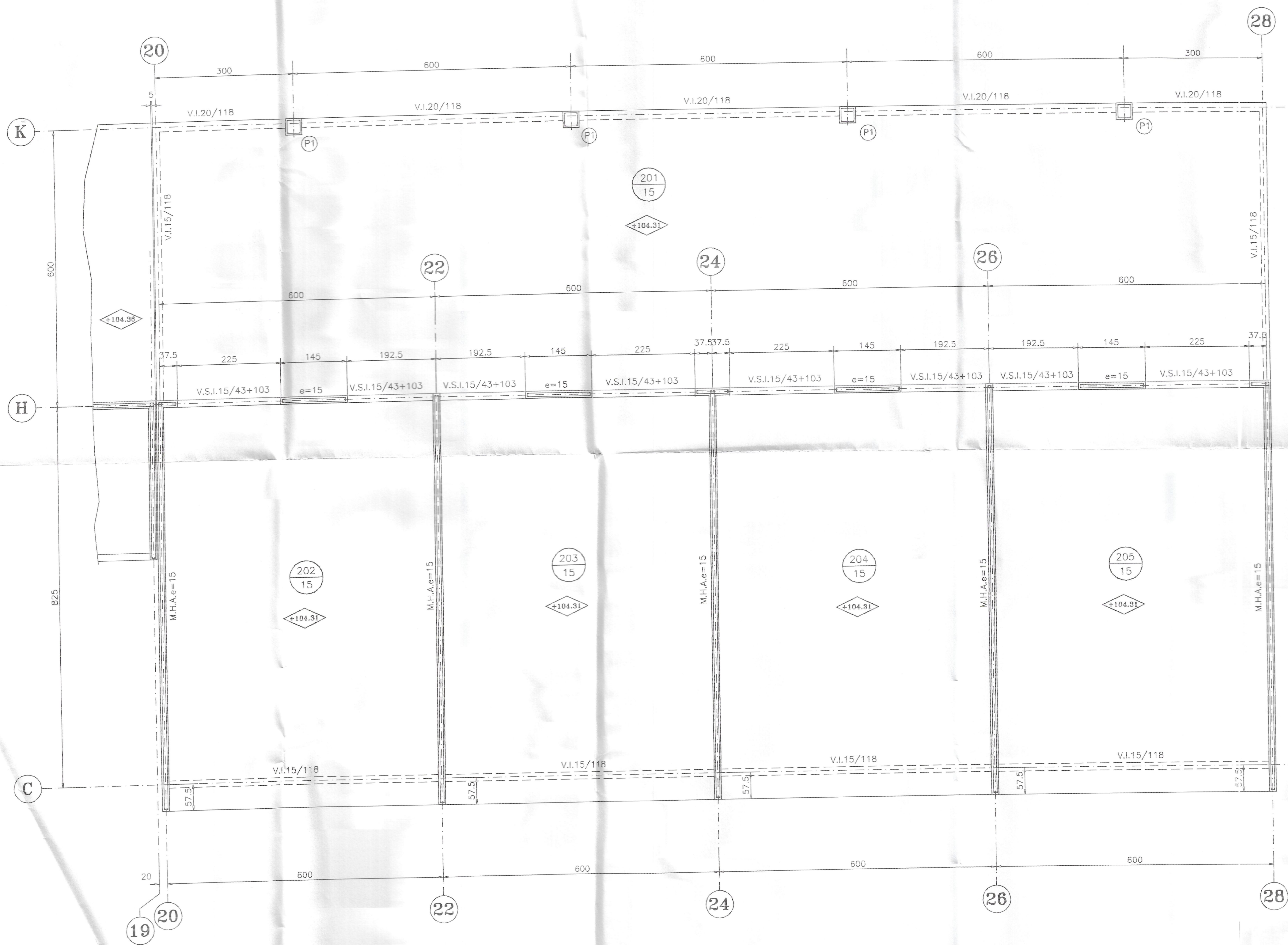
PLANTA DE ESTRUCTURAS 2ºPISO ESCALA 1:50
