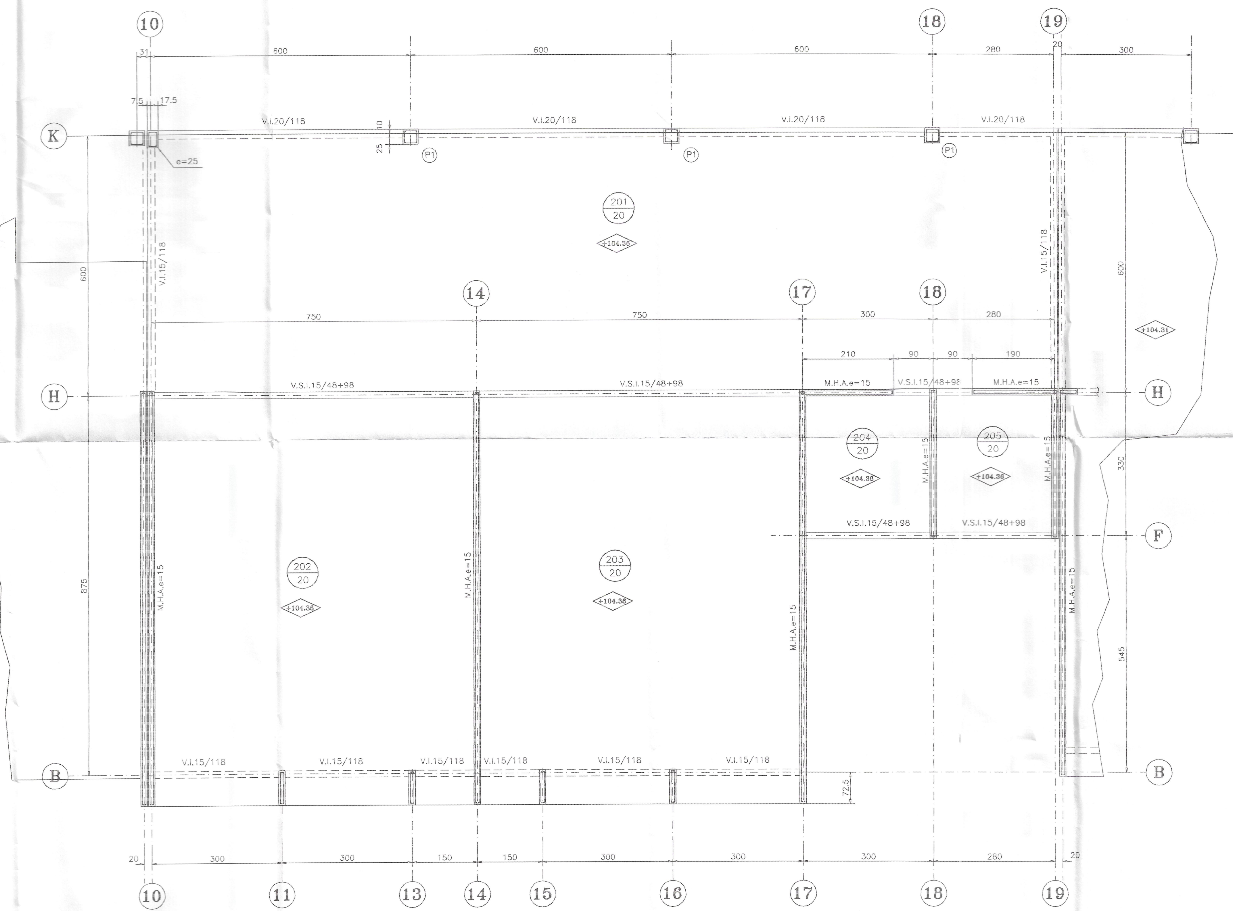
PLANTA DE ESTRUCTURAS 2ºPISO ESCALA 1:50
