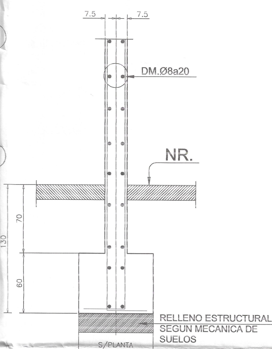
CORTE FUNDACION TIP. ESC. 1:20
