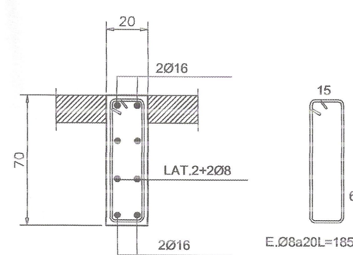
VF. 20/70 ESC. 1:20
