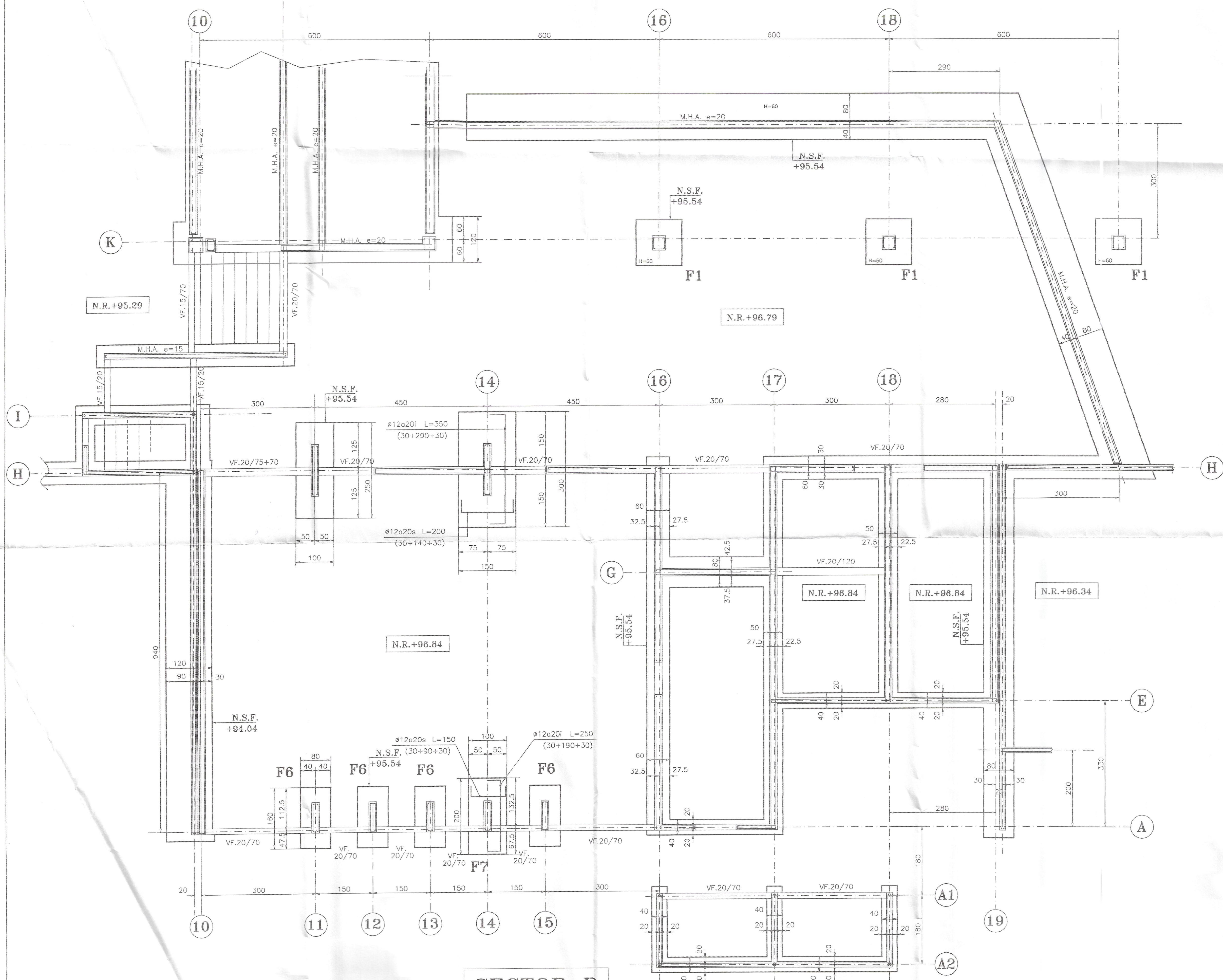
PLANTA DE FUNDACIONES ESCALA 1:50
