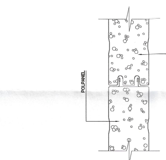
DETALLE UNION DE PANELES
