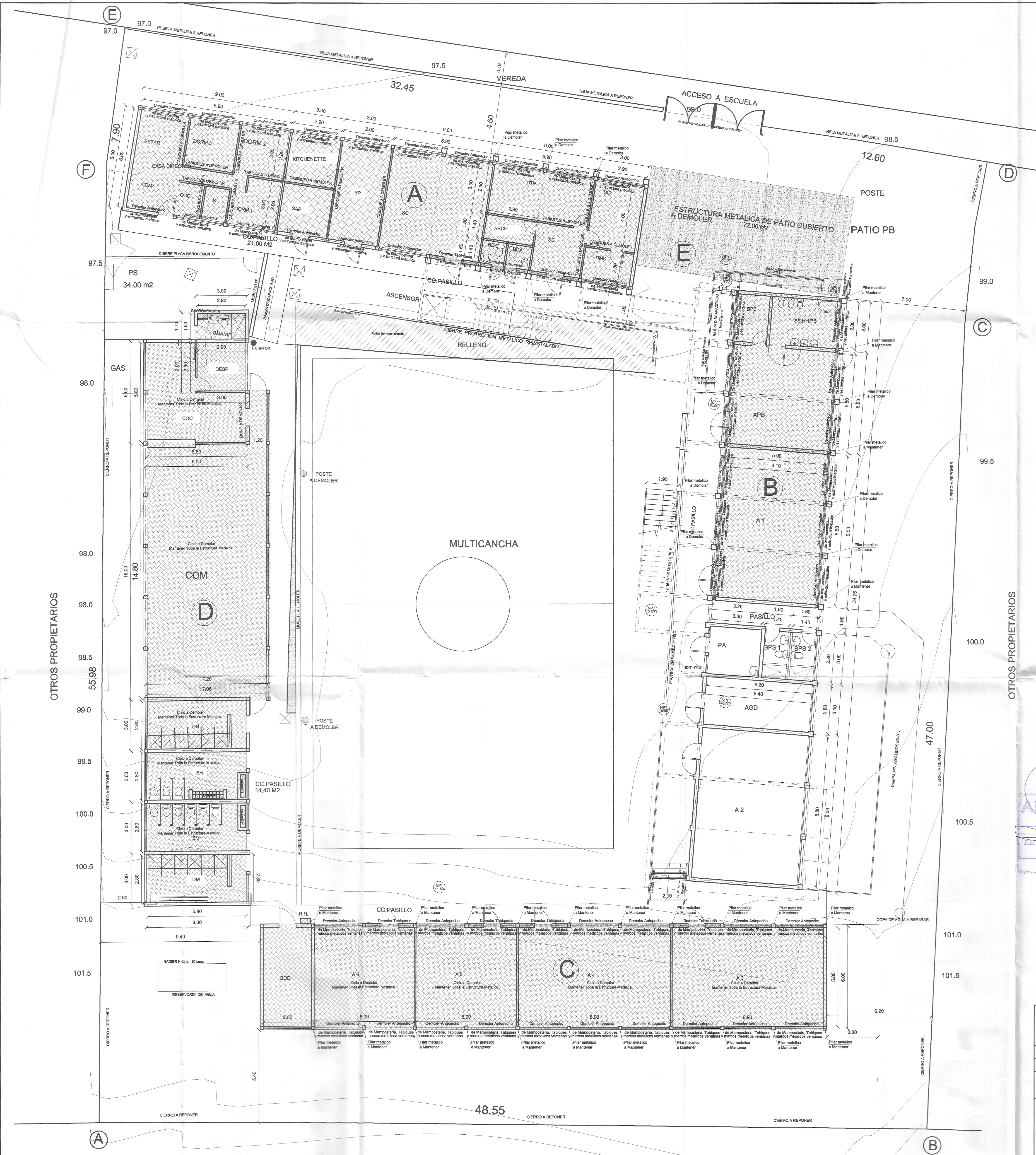
PLANTA EMPLAZAMIENTO DE DEMOLICION Y REPARACIONES ESCALA 1:100
