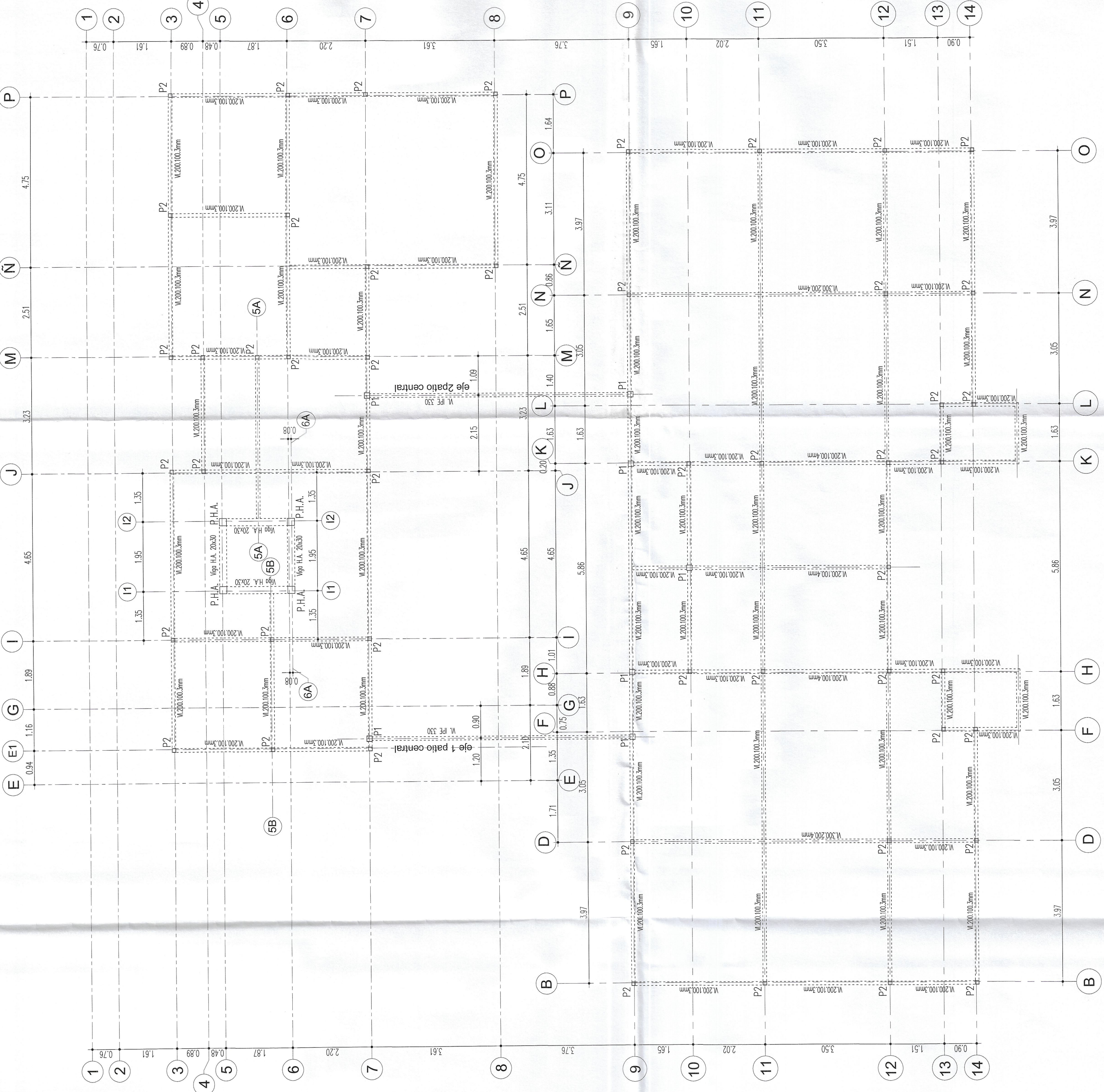
PLANTA DE ESTRUCTURA 2º PISO
